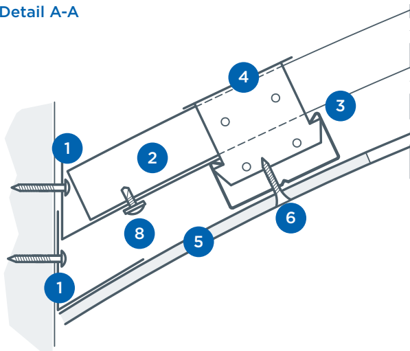
Detail A-A
